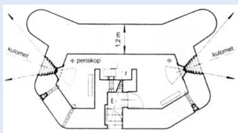
Řez pevnůstkou
